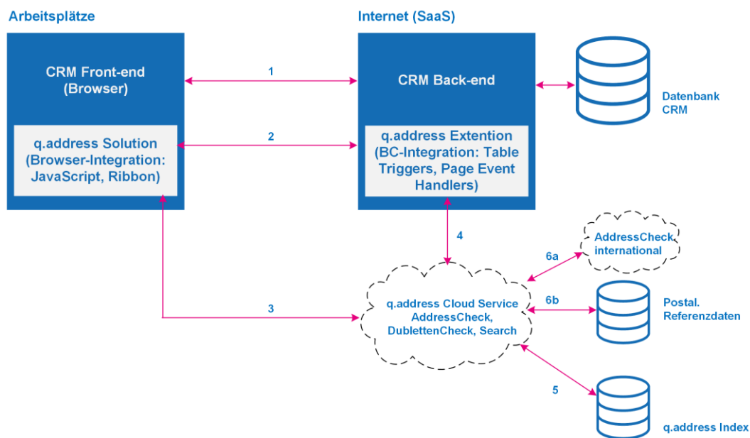
Bild 3: Architektur q.address Add-on SaaS für Dynamics 365 Business Central.
