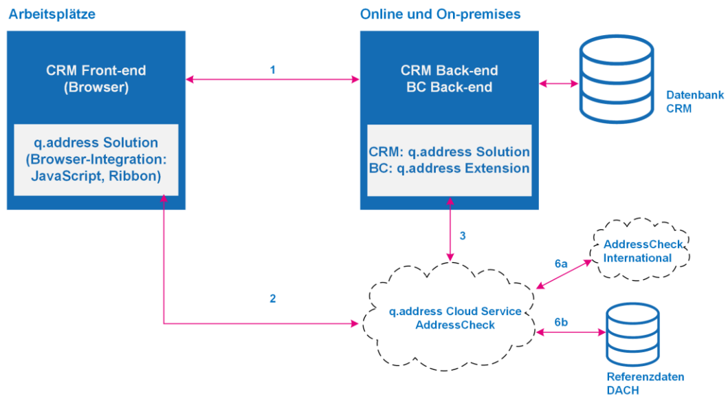
Bild 1: Architektur q.address AddressCheck SaaS für Dynamics 365 CRM und BC Online und On-premises.
