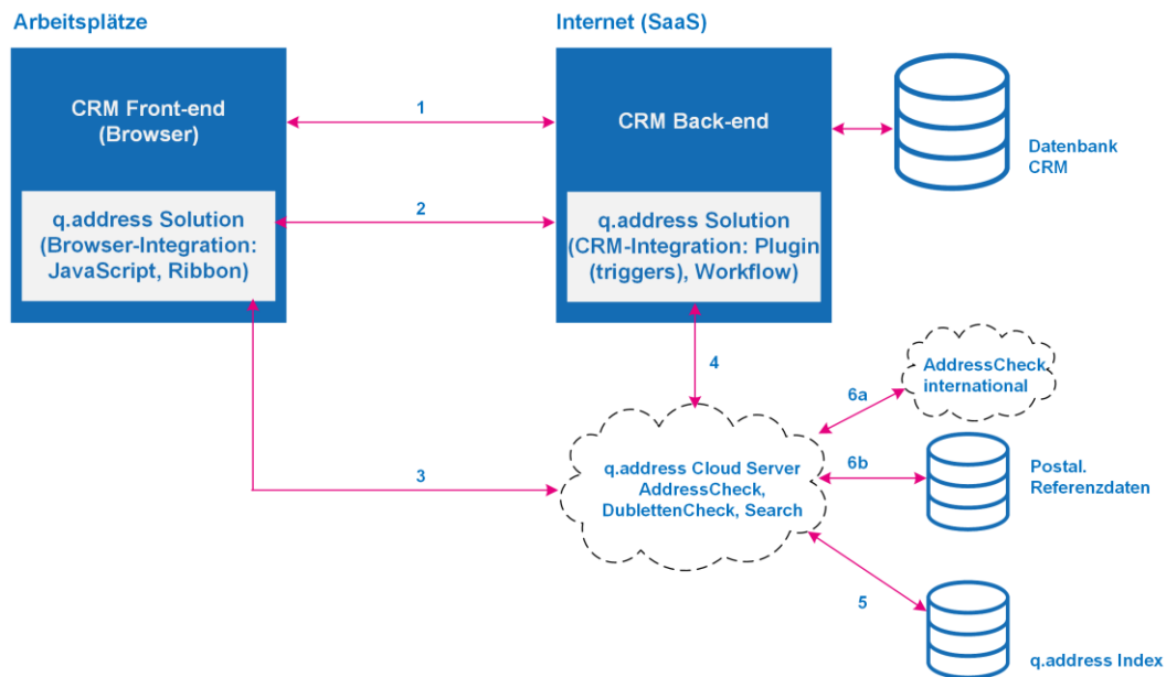
Bild 2: Architektur q.address Add-on SaaS für Dynamics 365 CRM.
